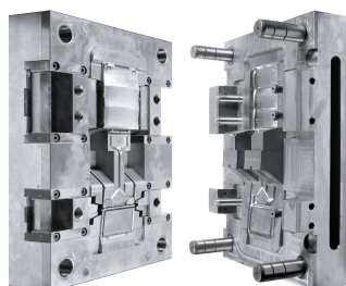
Spritzgießform „Wrangler-Jeep“ von Weiss Umformwerkzeuge
